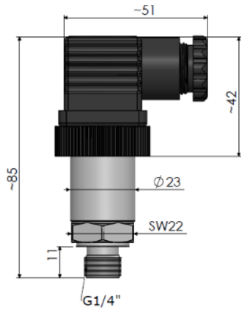
S30: DIN43650-A CONNECTOR
