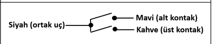
Kablo Çıkışı
